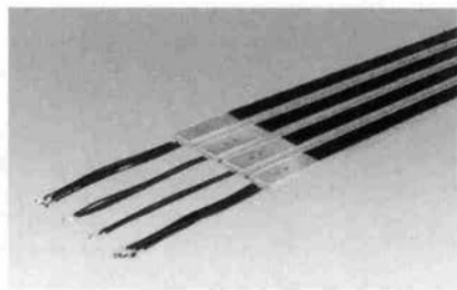
車両検知センサー 有料道路の路面に埋設し、ETCなど通過車両の車種判別に使われるセンサー。高速道路網の整備にともなって、ますます需要が見込まれる。
