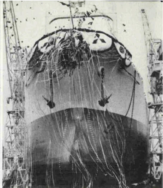
強風下で進水した「シルバーロングェビティ」(1968.9.14)
