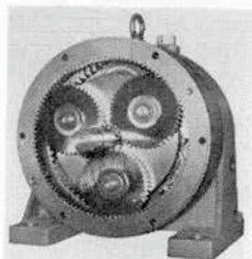
遊星減速機 (プラネタリー形)
