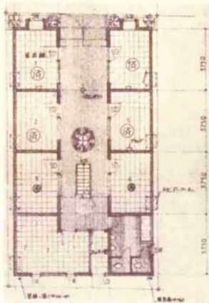
平面図1F
