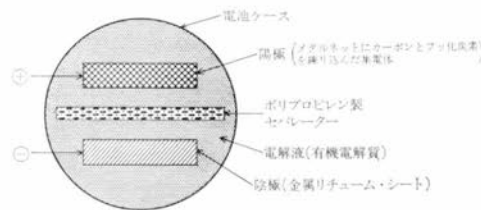
有機電解質リチウム電池の概念図
