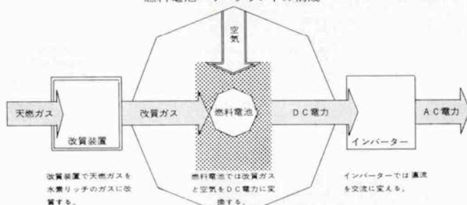
燃料電池パワープラントの構成
