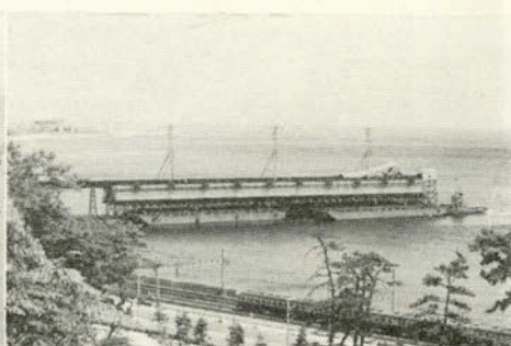
▲ベルトコンベアとプッシャーバージ
