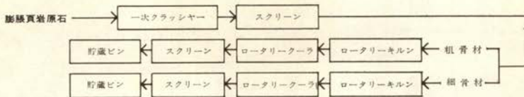
非造粒型膨脹頁岩骨材の製造工程
